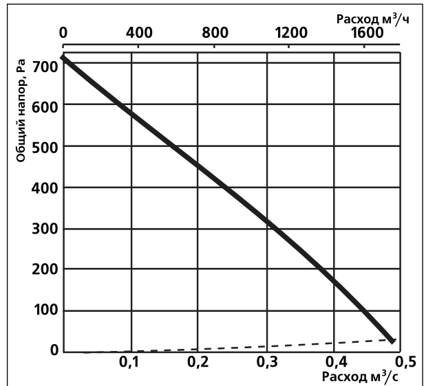
Канал-ВЕНТ-315В
