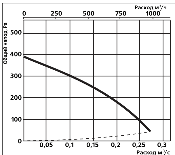
Канал-ВЕНТ-200А
