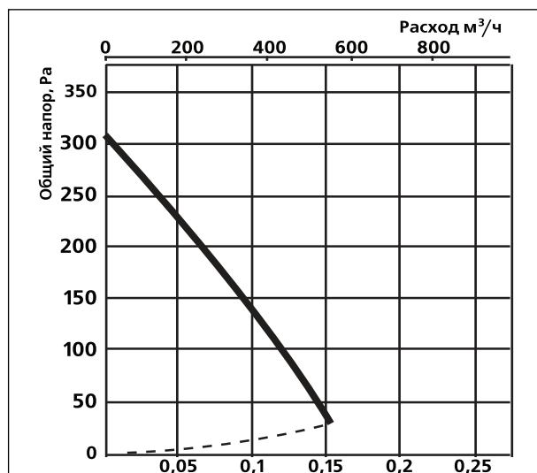
Канал-ВЕНТ-200В
