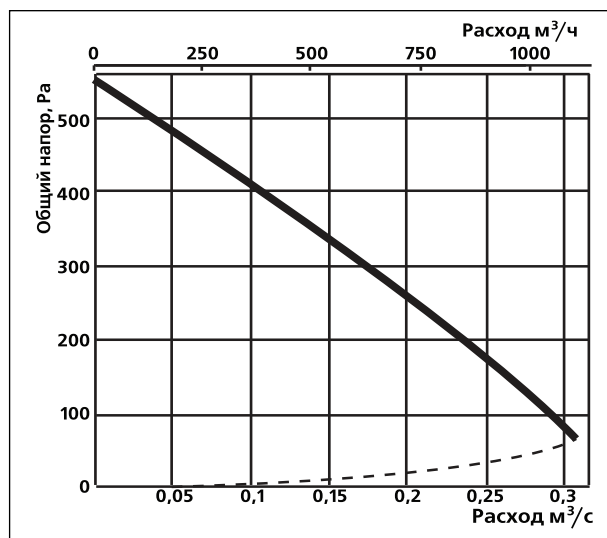
Канал-ВЕНТ-200В
