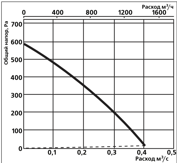
Канал-ВЕНТ-315А
