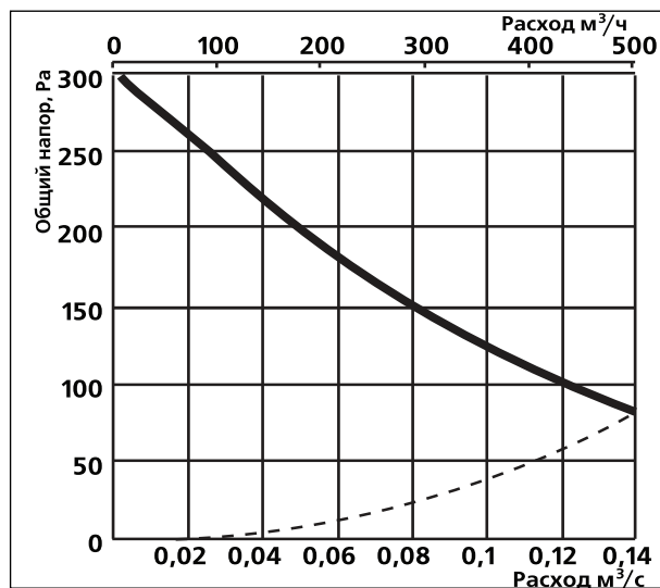
Канал-ВЕНТ-160А
